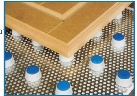
RAPHA Jig Pinsystem Typ "STARTER"
